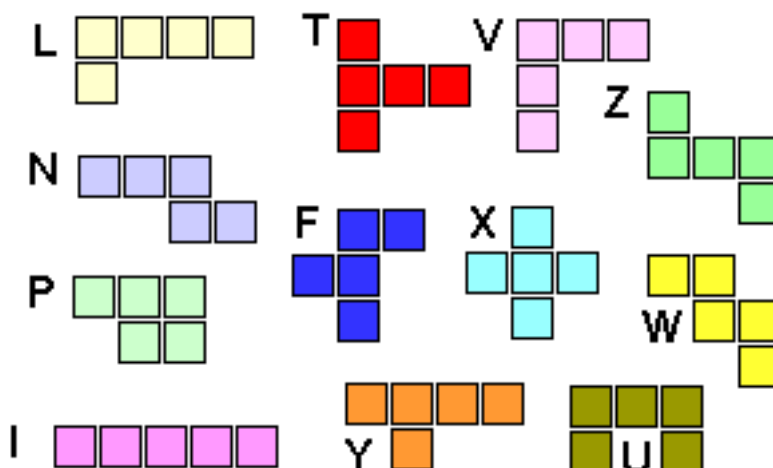
Les douze pentaminos, composés chacun de 5 cases.
